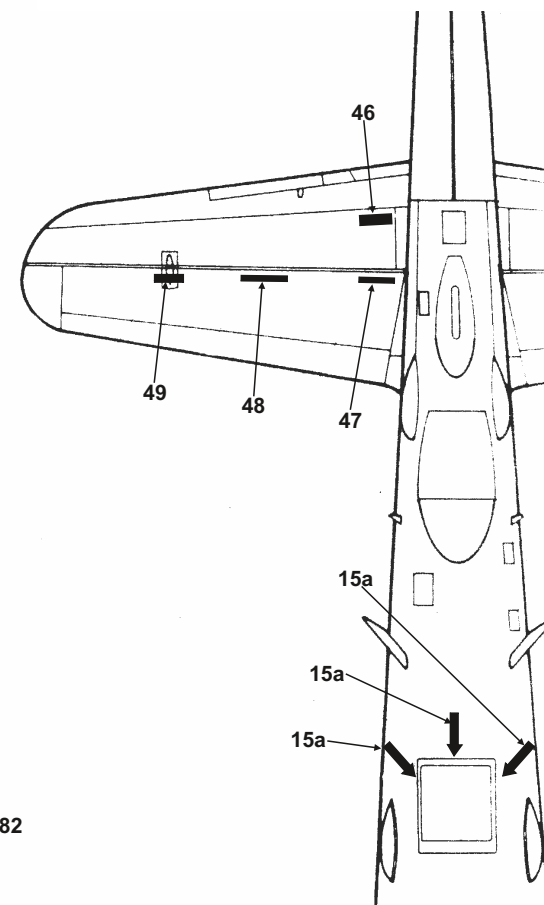
Spodní strana výškovky - stejné pro obě strany Bottom side of the elevator - same for both sides
