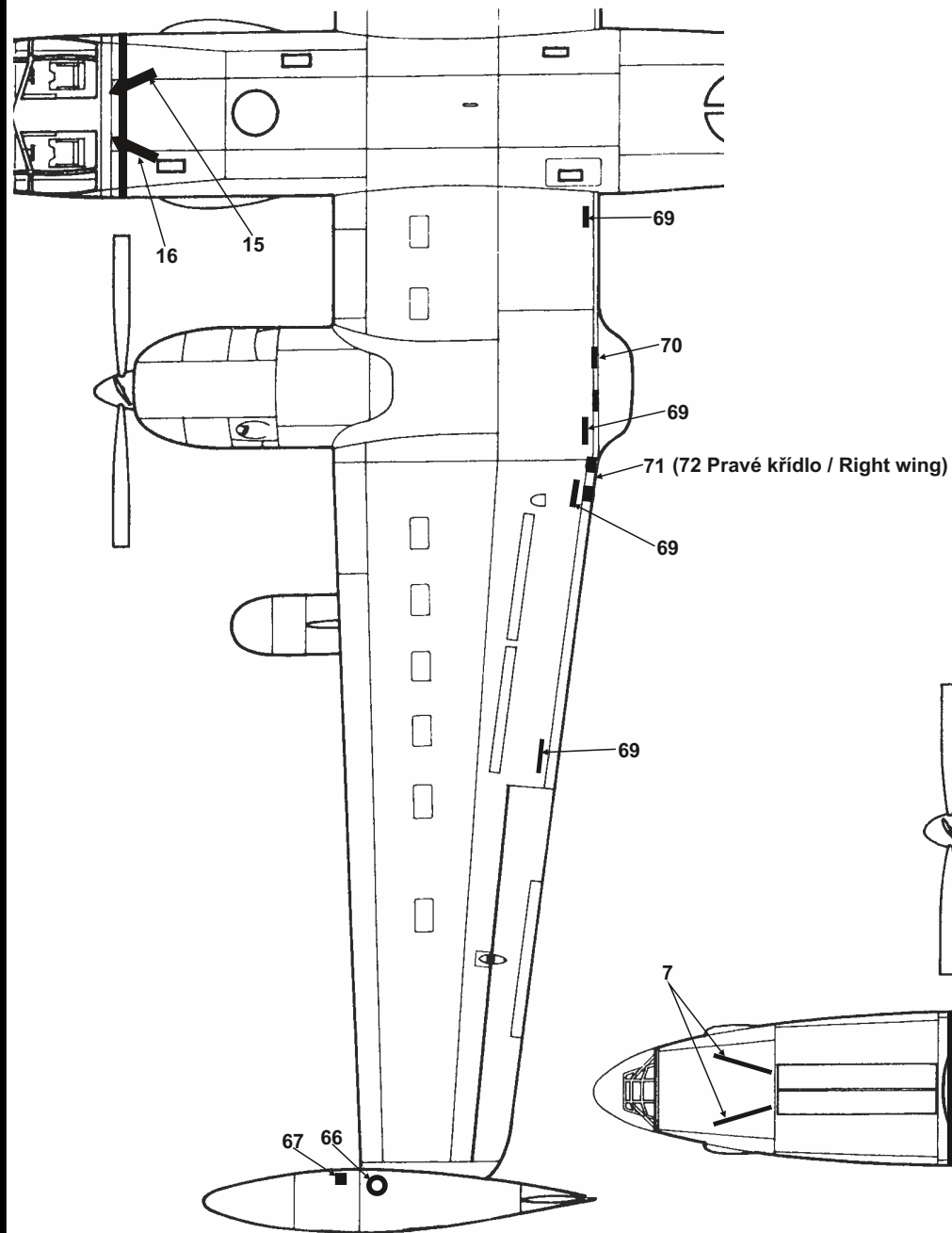
Vrchní strana křídel - stejné pro levé i pravé křídlo Top side of the wings - same for both wings
